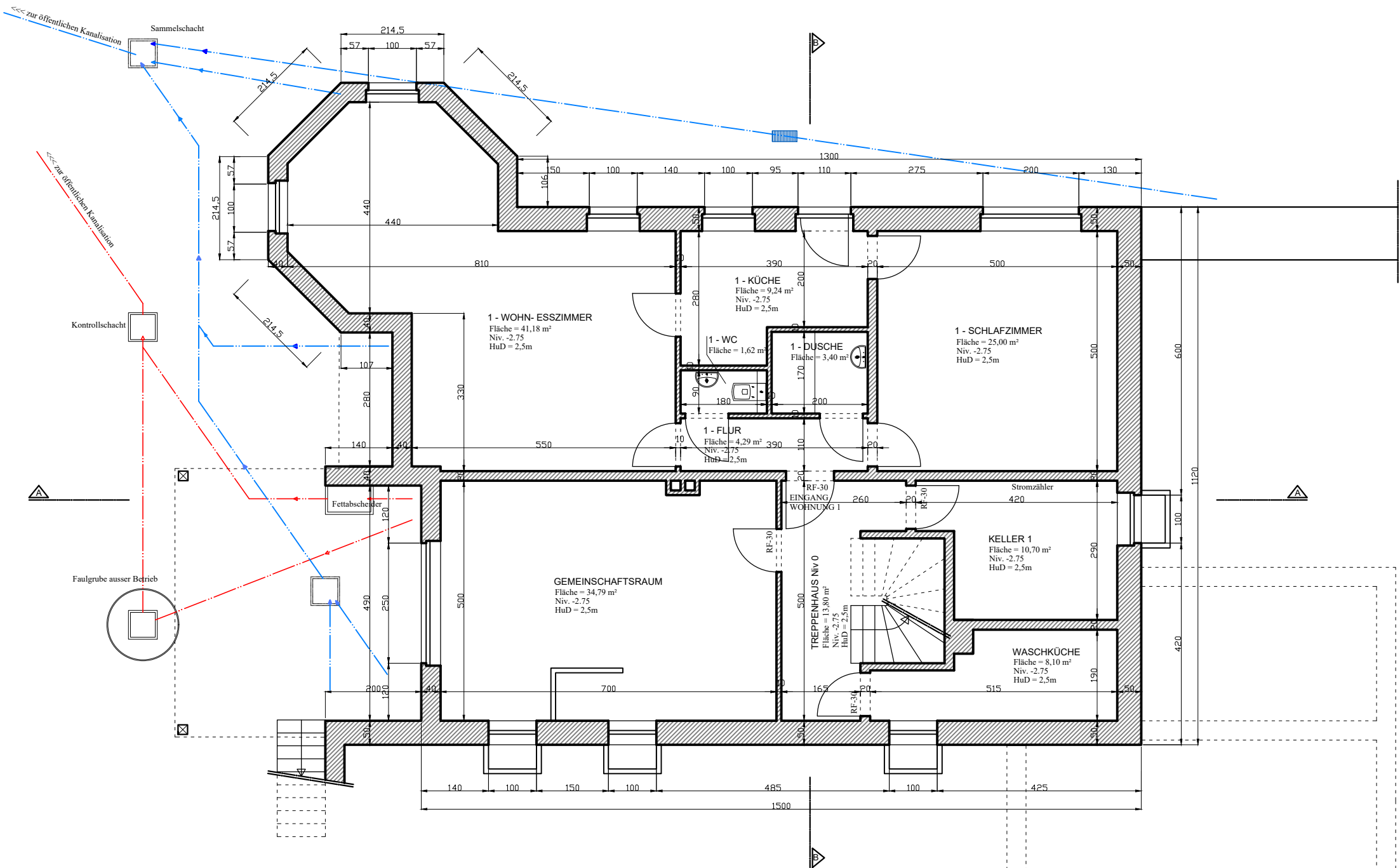
KELLERGESCHOSS 1/100
